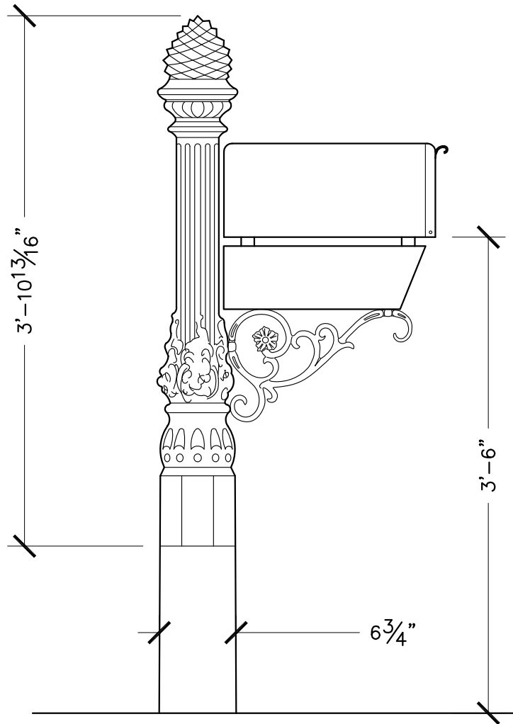
ELEVATION
