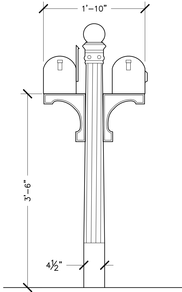
ELEVATION
